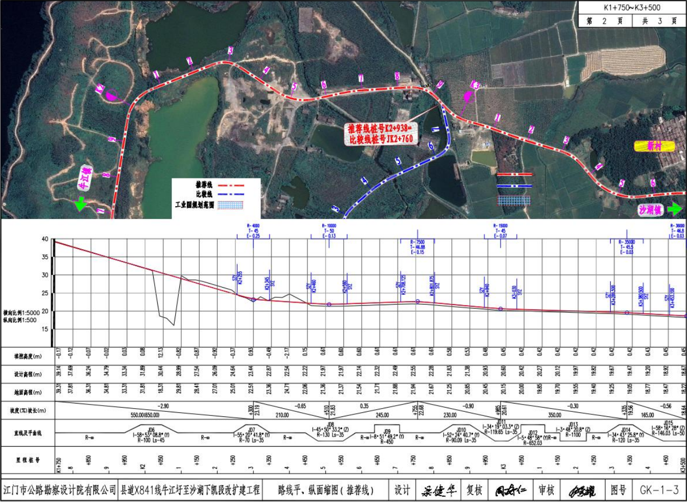
图 2-2 路线平、纵缩图（b）
