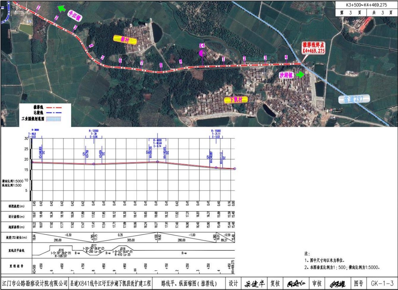
图 2-3 路线平、纵缩图 (c)
