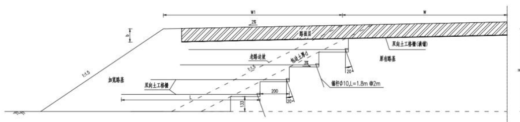
图2-4 新旧路基拼接示意图
