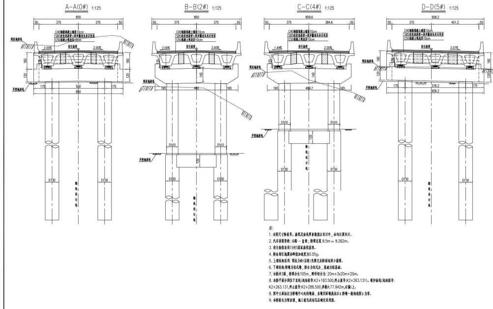
图2-7b K2+236.0泄洪渠1号桥桥型总体布置图
