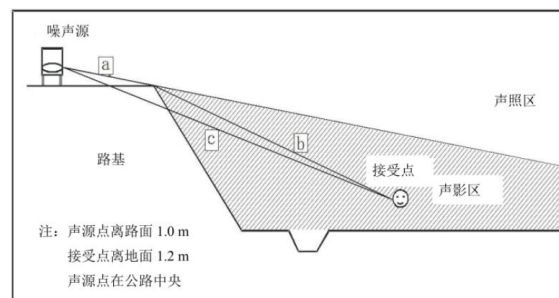
图 4-8 声程差 \delta 计算示意图
