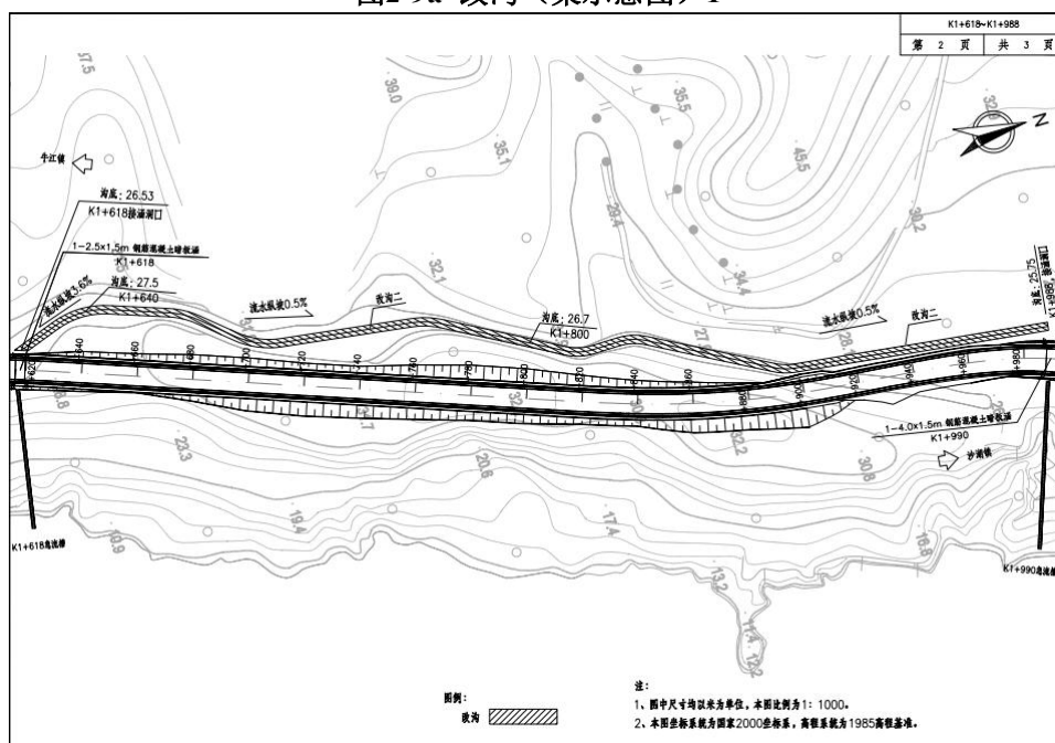
图2-9b 改沟（渠示意图）2
