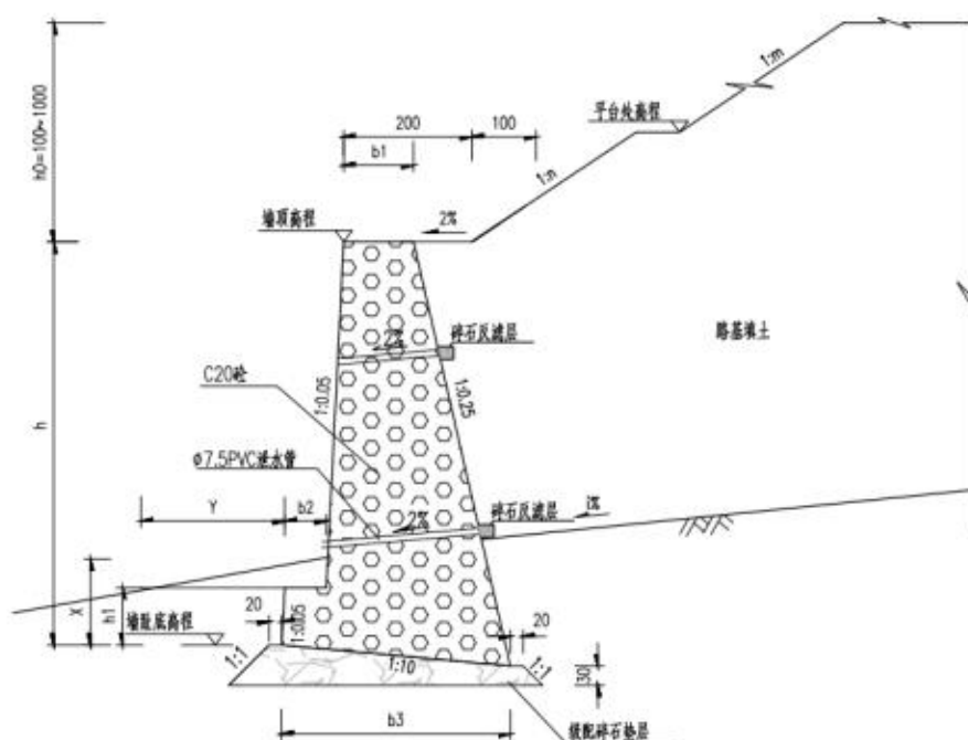
图2-5 挡土墙示意图
