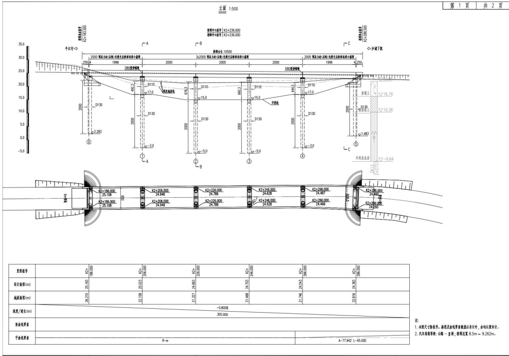
图2-7a K2+236.0泄洪渠1号桥桥型总体布置图
