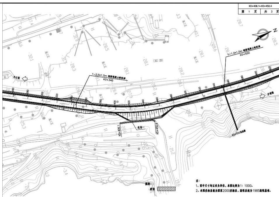
图2-9a 改沟（渠示意图）1
