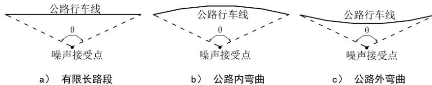
图 4-1 预测点到有限长路段两端的张角
