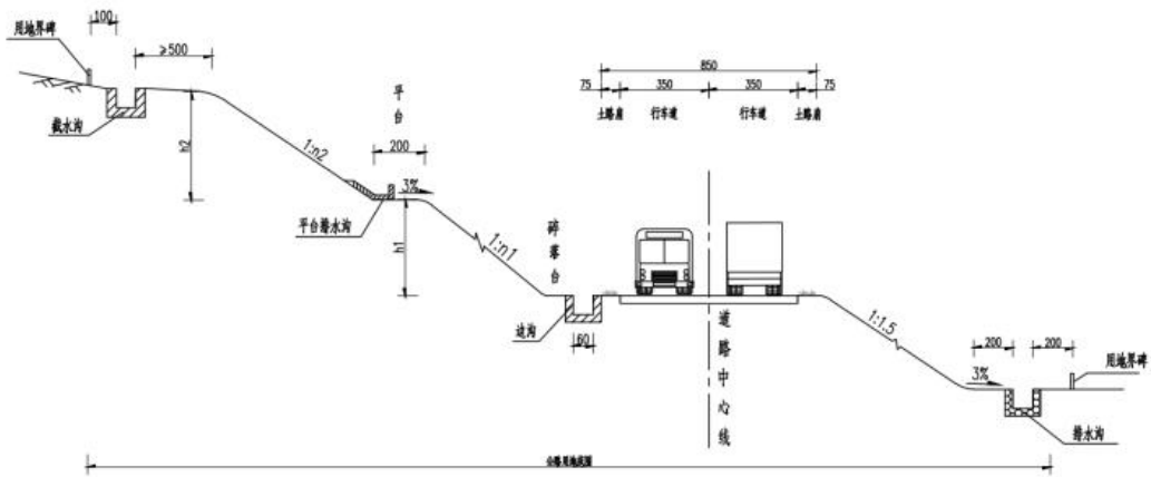
图2-3 改扩建后路基标准横断面图
