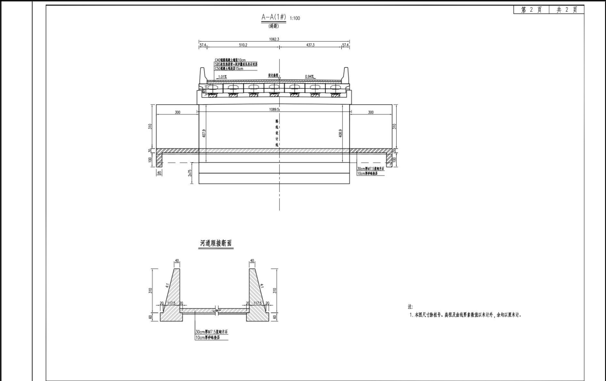
图2-8b K2+586.0泄洪渠2号桥桥型总体布置图
