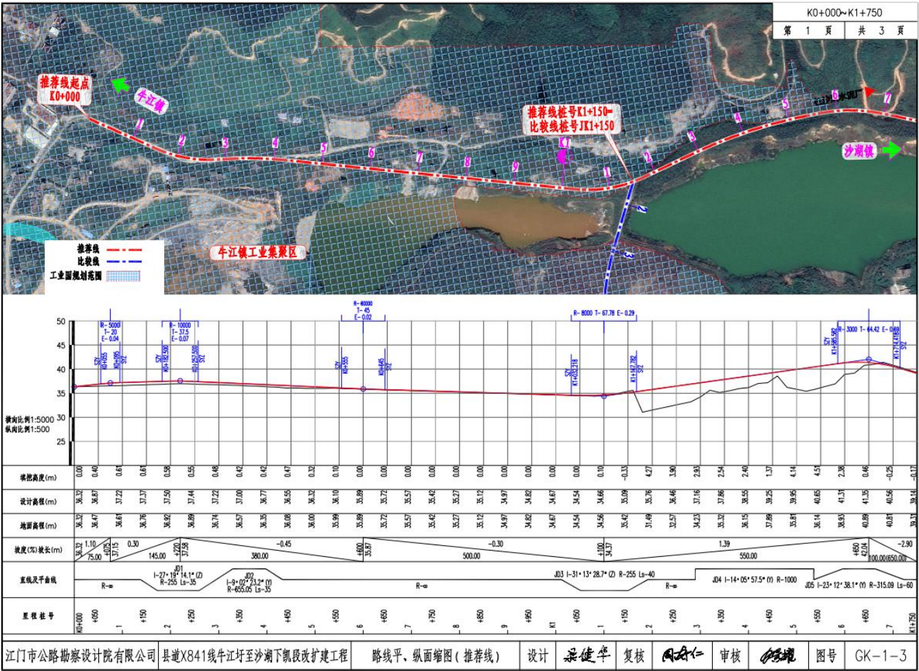
图 2-1 路线平、纵缩图 (a)
