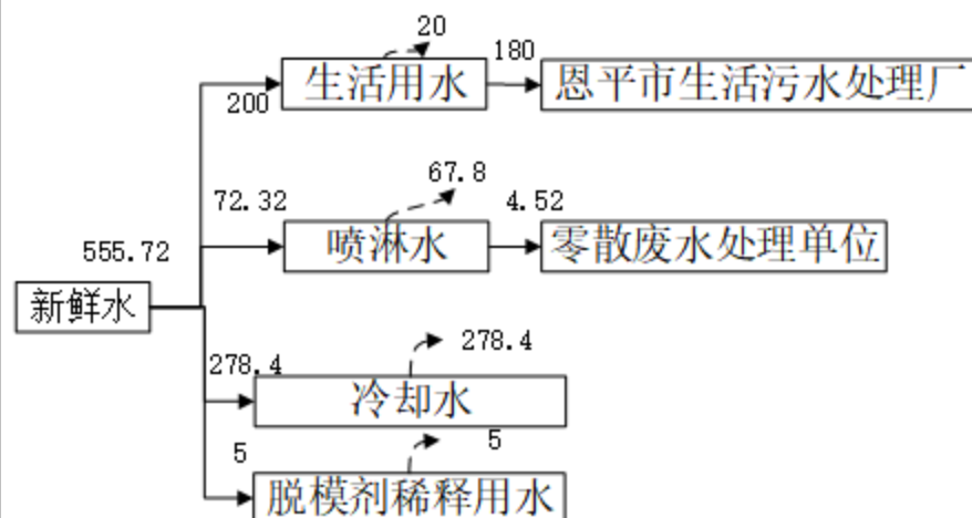
图 2-1 项目水平衡图（单位：m³/a）
