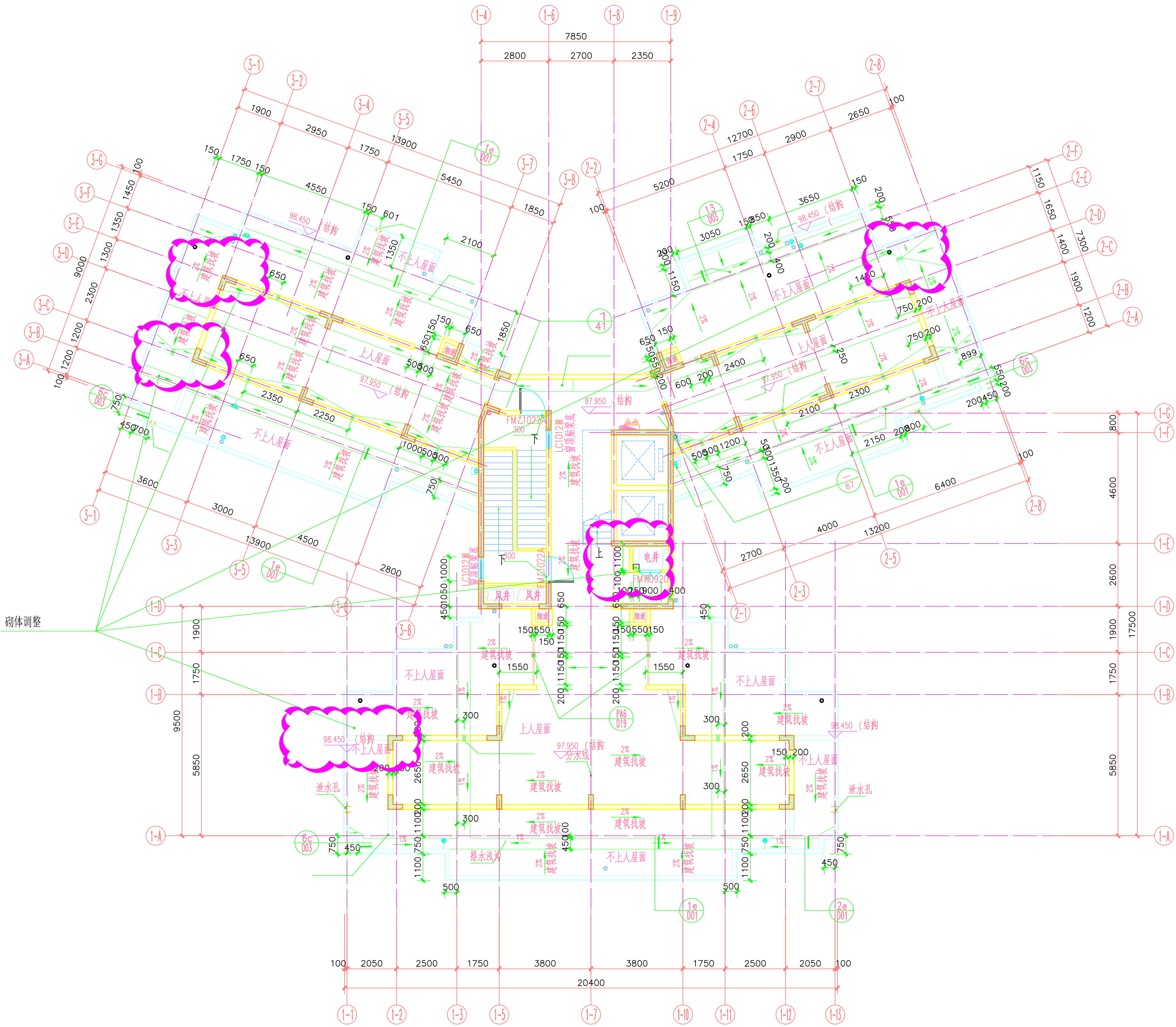
屋顶层平面图 1:100
