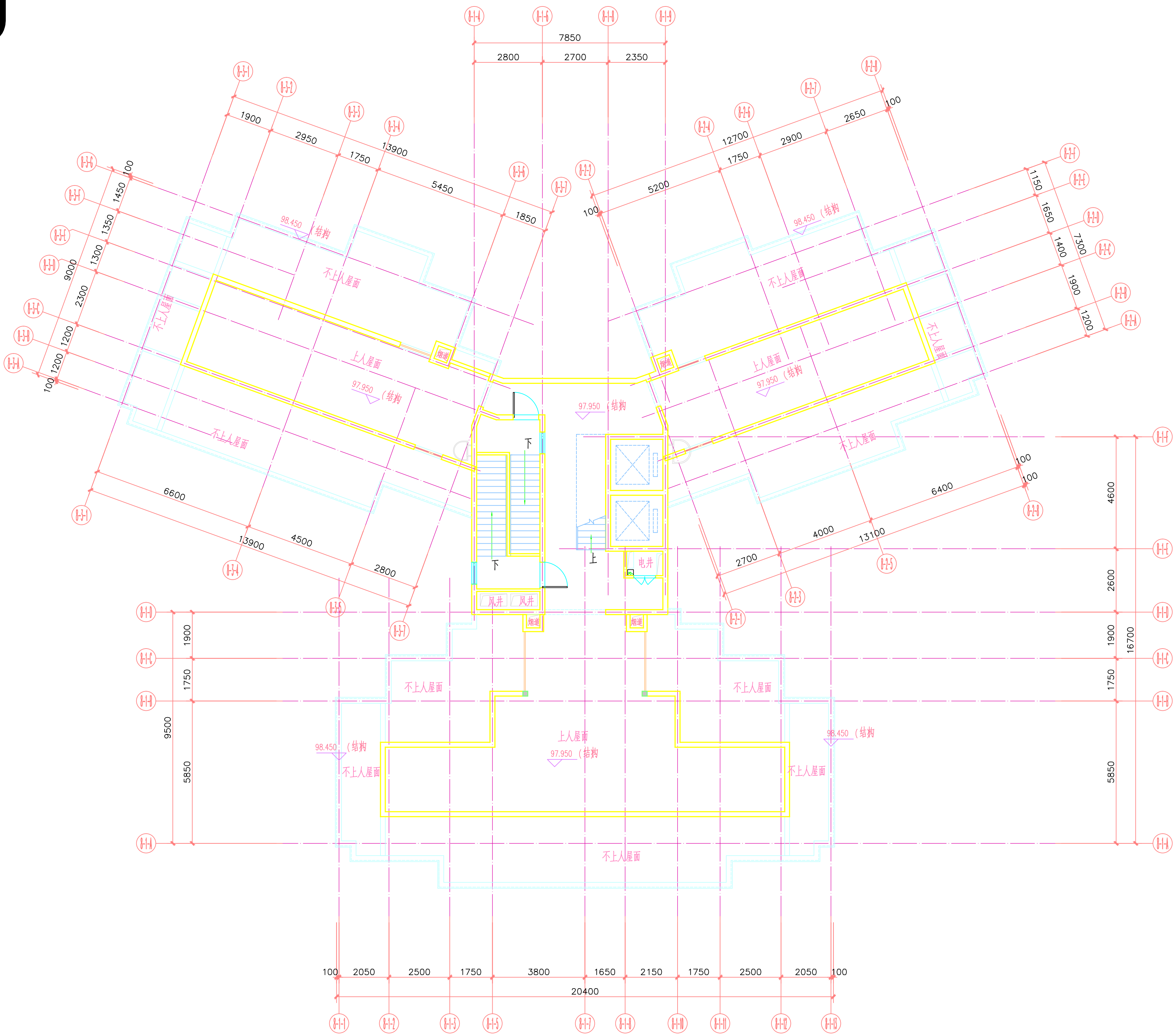
屋面层平面图 1:100
