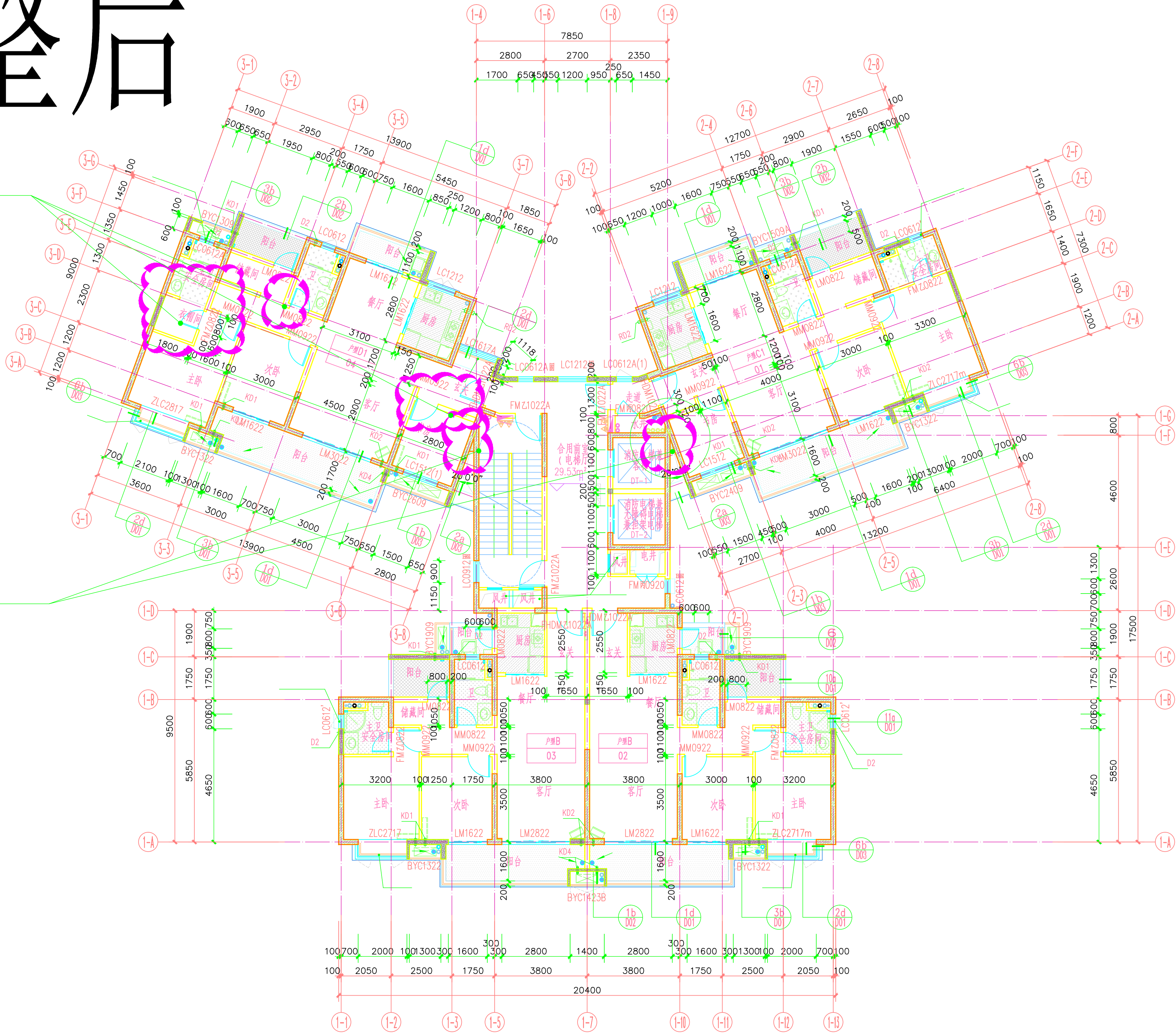
四~三十三层平面图 1:100
